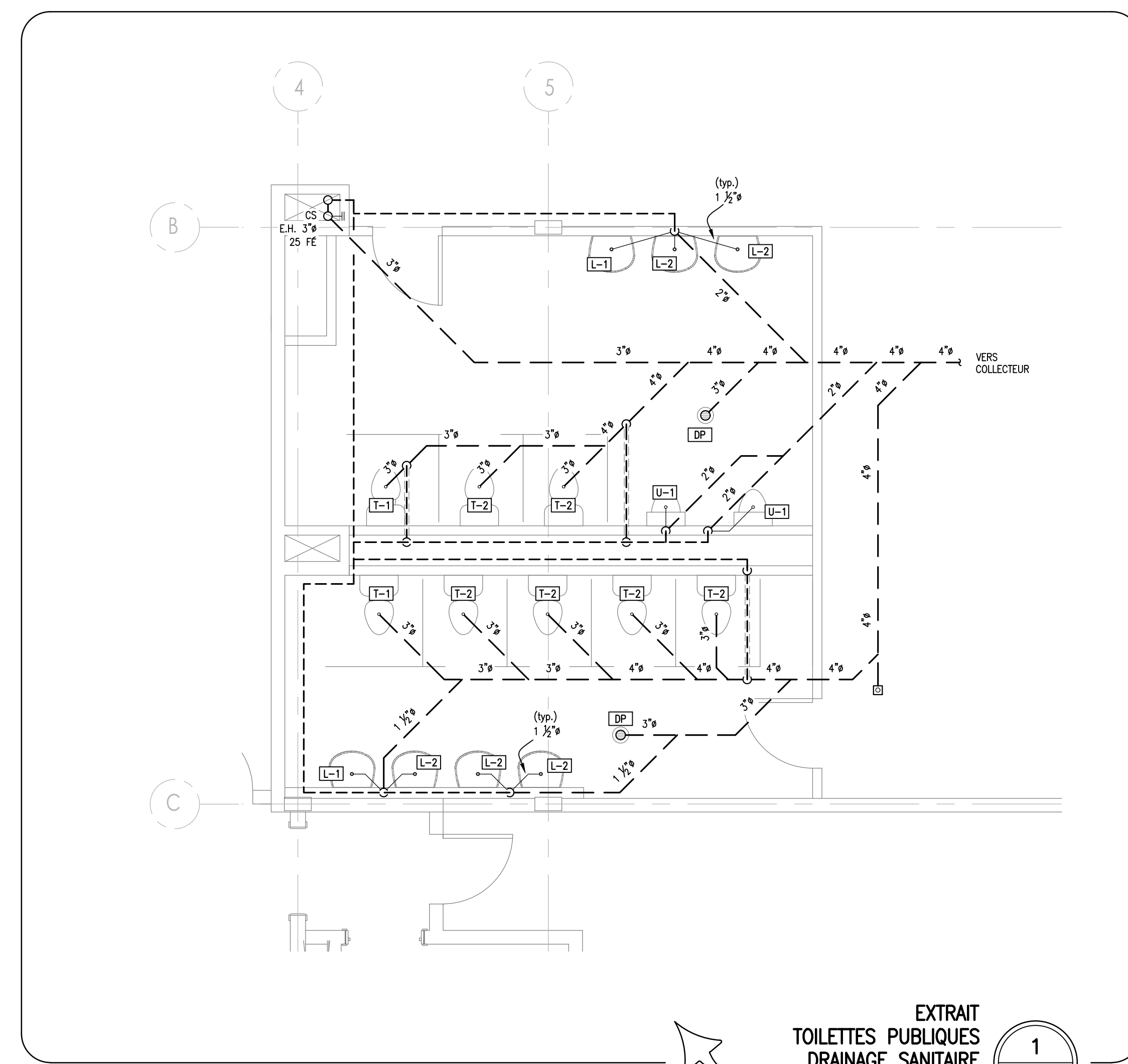
DIAGRAMME DRAINAGE SANITAIRE ECHELLE: AUCUNE
