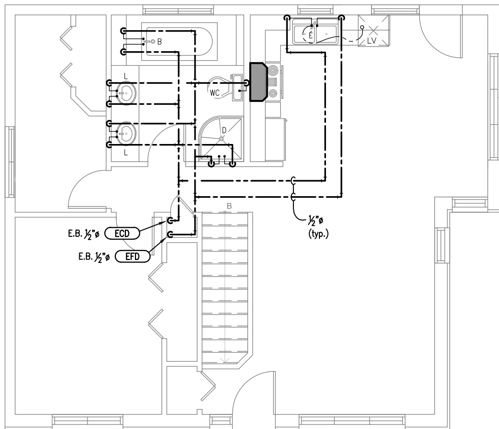
PLAN REZ-DE-CHAUSSÉE
