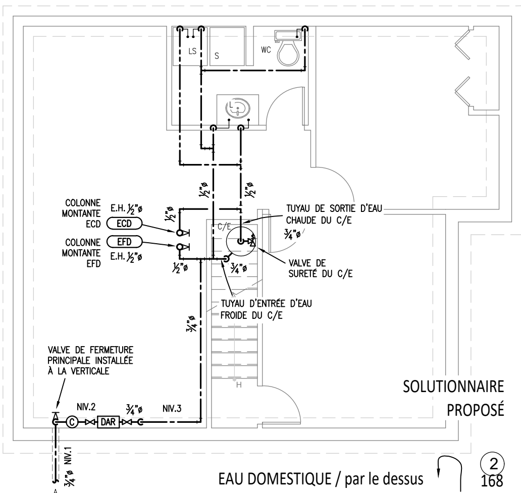
PLAN SOUS-SOL
